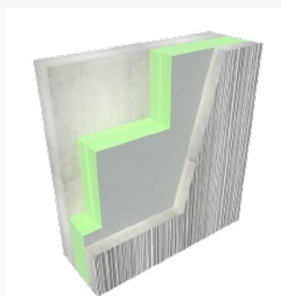
PREFABRYKOWANA TRÓJWARSTWOWA ŚCIANA BETONOWA ZBROJONA
