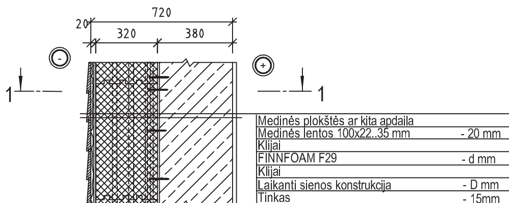
Pjūvis 1-1
