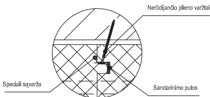
Detalė A Mastelis 1:5
