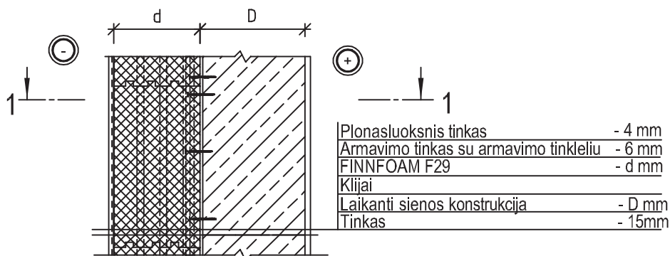
Pjūvis 1-1
