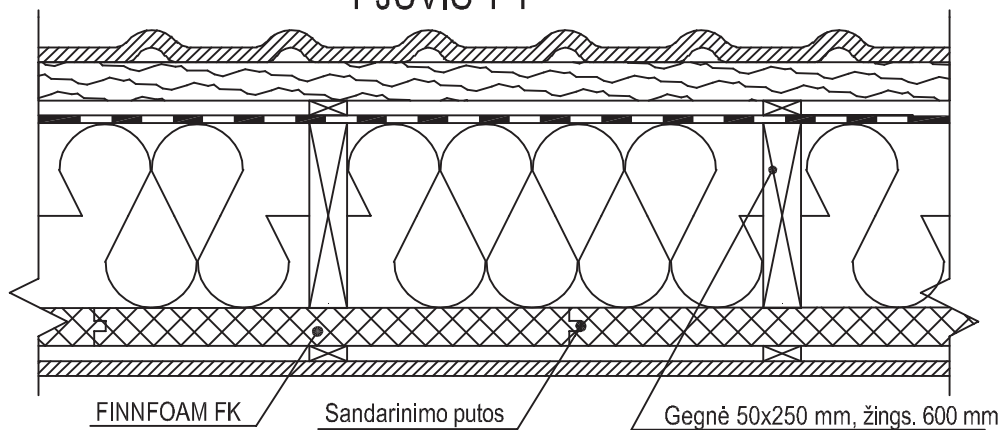
PJŪVIS 1-1
